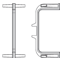
81/G13.A90A 90° EXTERIOR
